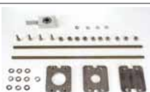
Positive Stops — механические концевые выключатели открывания/закрывания (встраиваемые в удлиненную модель привода 400)
